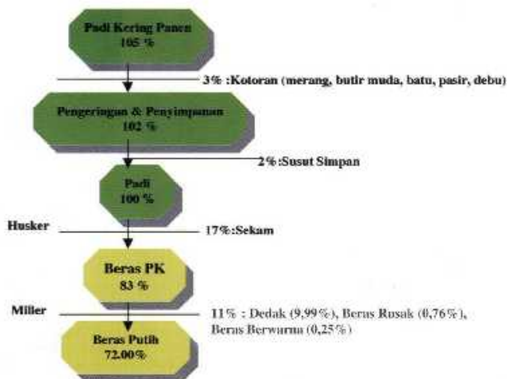
Gambar 3. Tahapan Utama Proses Pengolahan Beras
